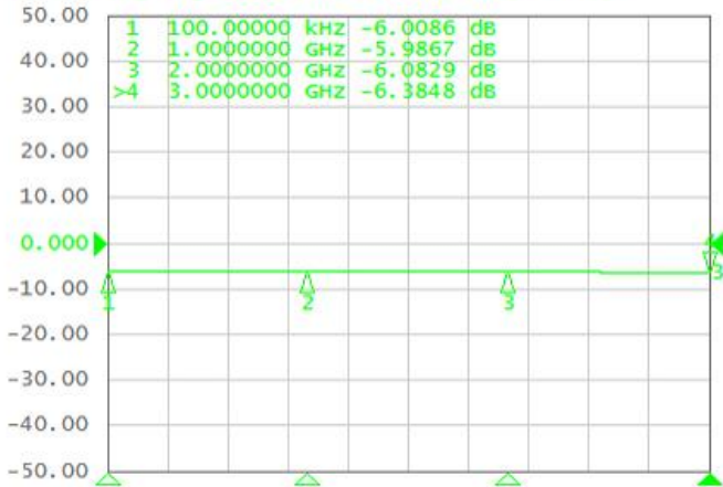
图3.隔离度
